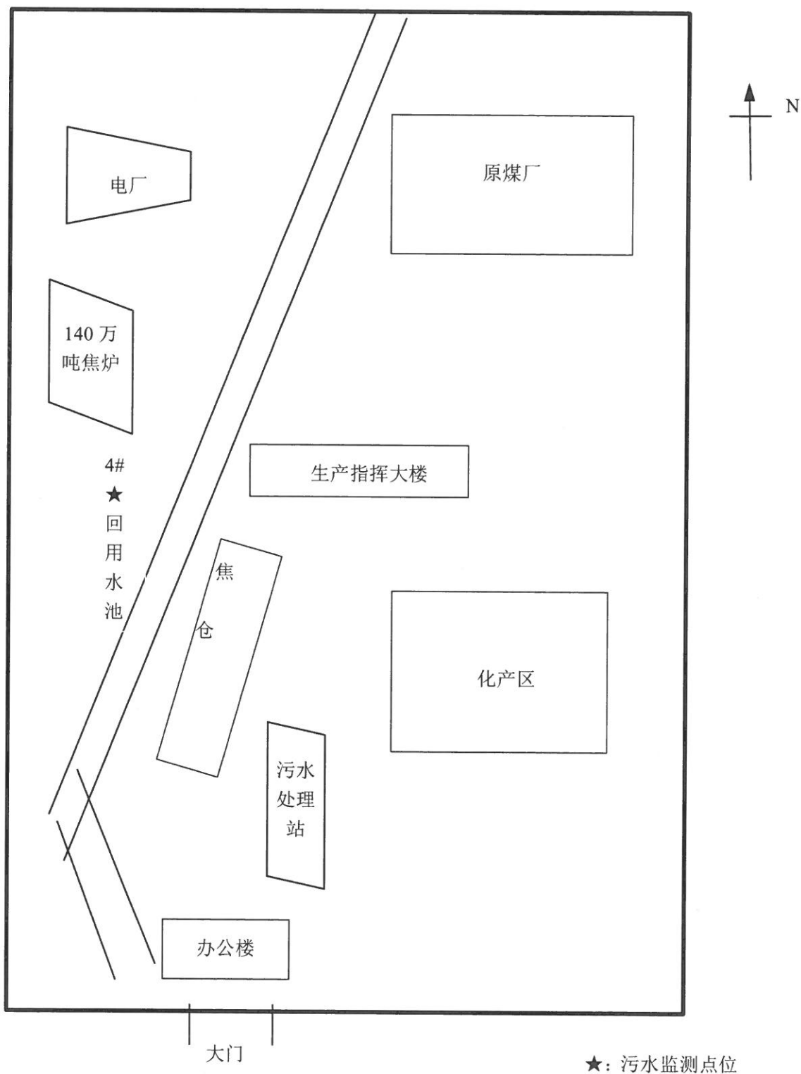
图 4-1 污水监测点位平面示意图
