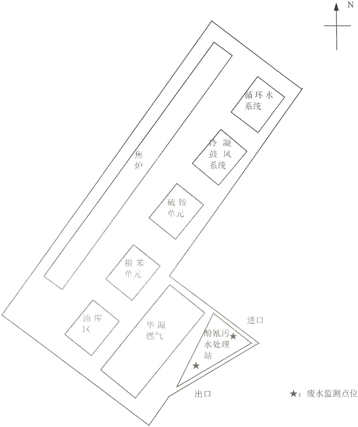
图 4-1 酚氰污水处理站监测点位平面示意图
